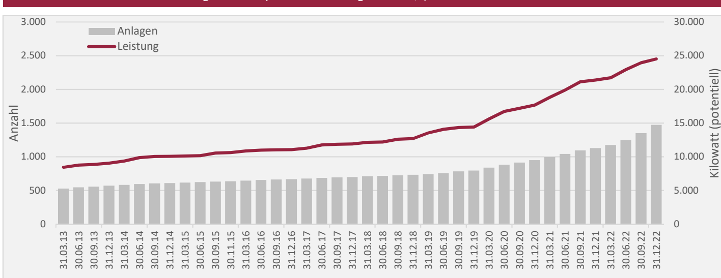
Abb. 3.13 Anzahl der Photovoltaik-Anlagen mit ihrer potentiellen Leistung in Koblenz, Quartale
