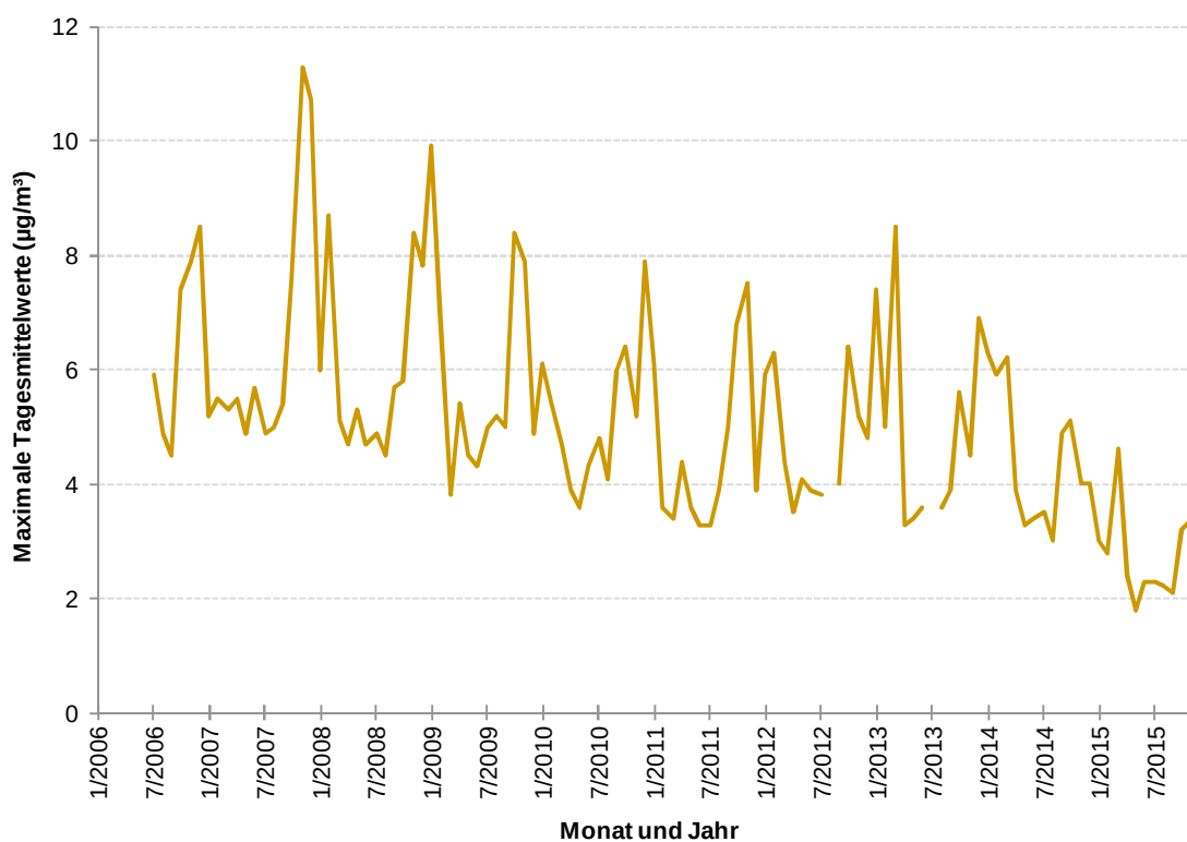
Abb. 3.04: Maximale Tagesmittelwerte der Belastung der Luft durch Rußpartikel in Koblenz (Messstelle Hohenfelder Straße)
