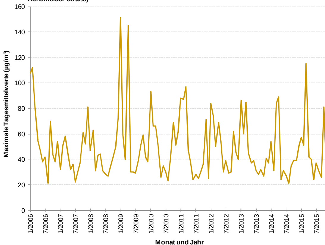
Abb. 3.06: Maximale Tagesmittelwerte der Belastung der Luft durch Feinstaub (PM10) ( \mu\text{g}/\text{m}^3 ) in Koblenz (Messstelle Hohenfelder Straße)
