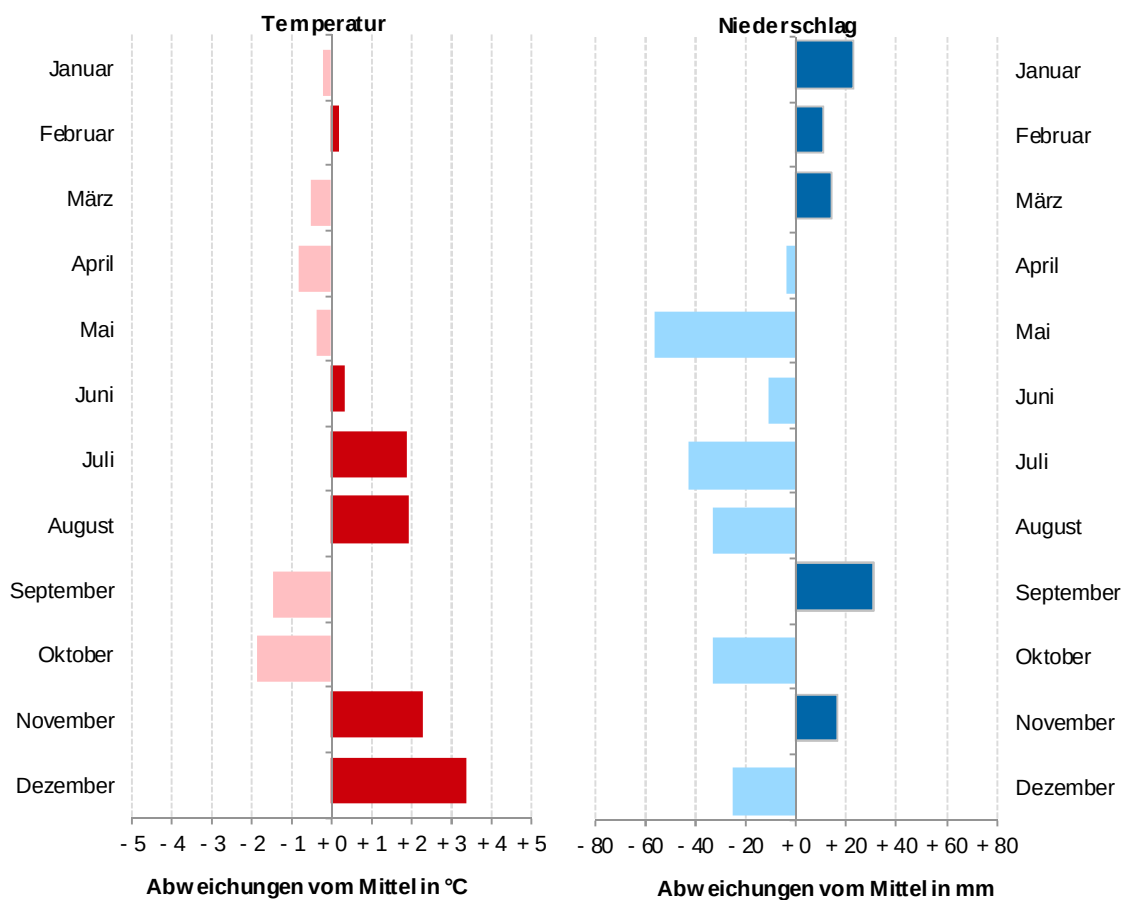
Abb. 3.02: Abweichung der monatlichen Niederschlagsmengen und Durchschnittstemperaturen 2015 vom Mittel der letzten fünf Jahre
